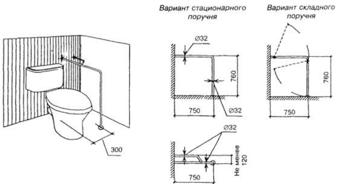
г — устройство двухопорного поручня при унитазах
