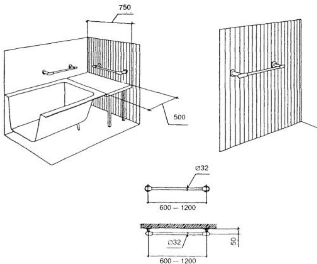
д — схема настенных поручней при ванне
