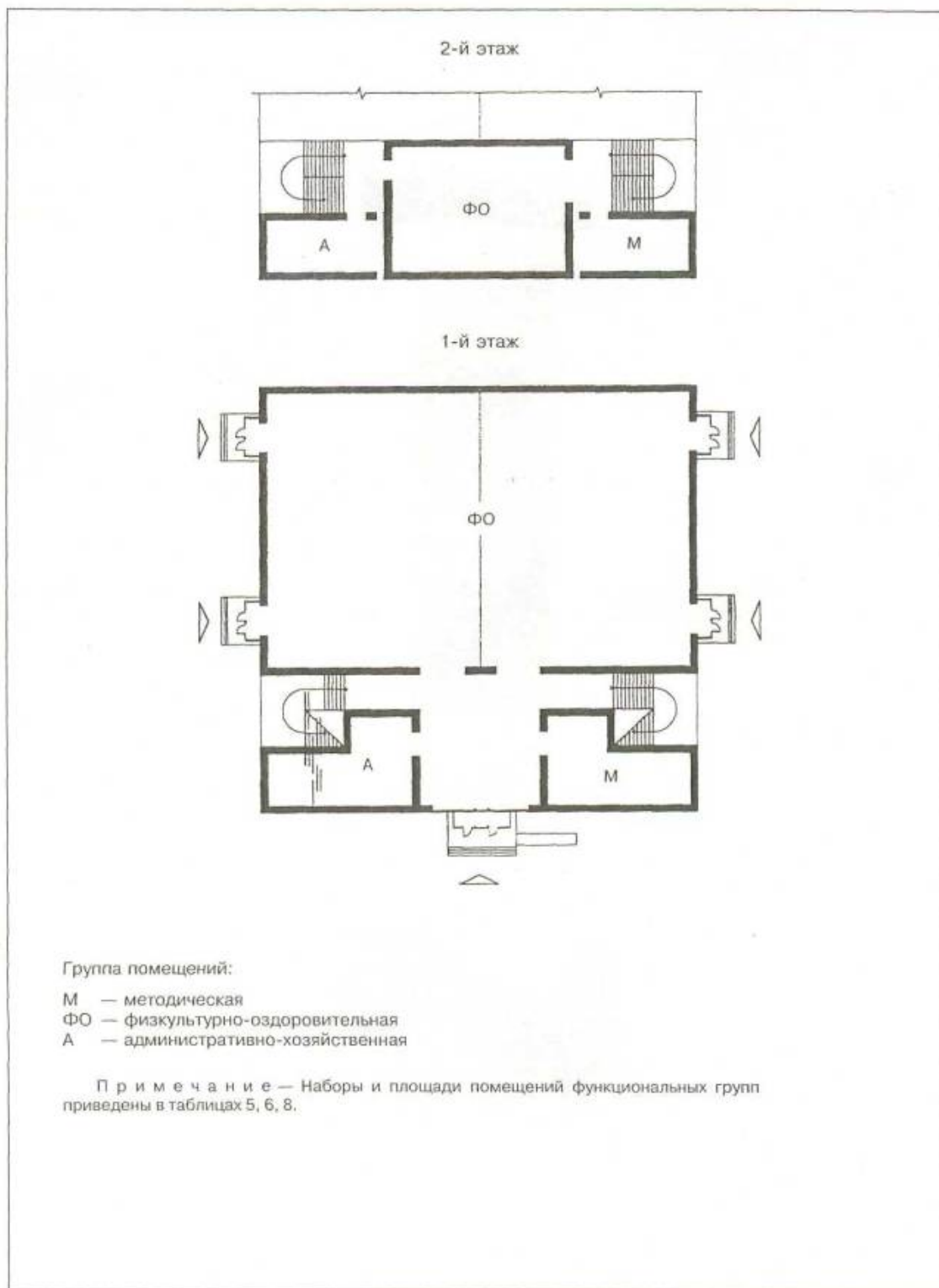
Рисунок Б.3 - Проектное решение консультационно-методического центра
