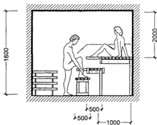
Разрез I—I
