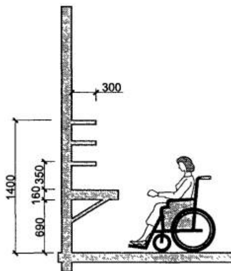
ГАБАРИТЫ УСТАНОВКИ ОБОРУДОВАНИЯ
