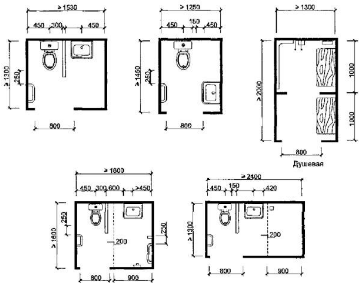
ОБОРУДОВАНИЕ САНИТАРНОГО УЗЛА С ДУШЕМ ДЛЯ ИНВАЛИДА НА КРЕСЛЕ-КОЛЯСКЕ
