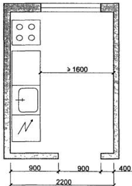
ГАБАРИТЫ УСТАНОВКИ ОБОРУДОВАНИЯ
