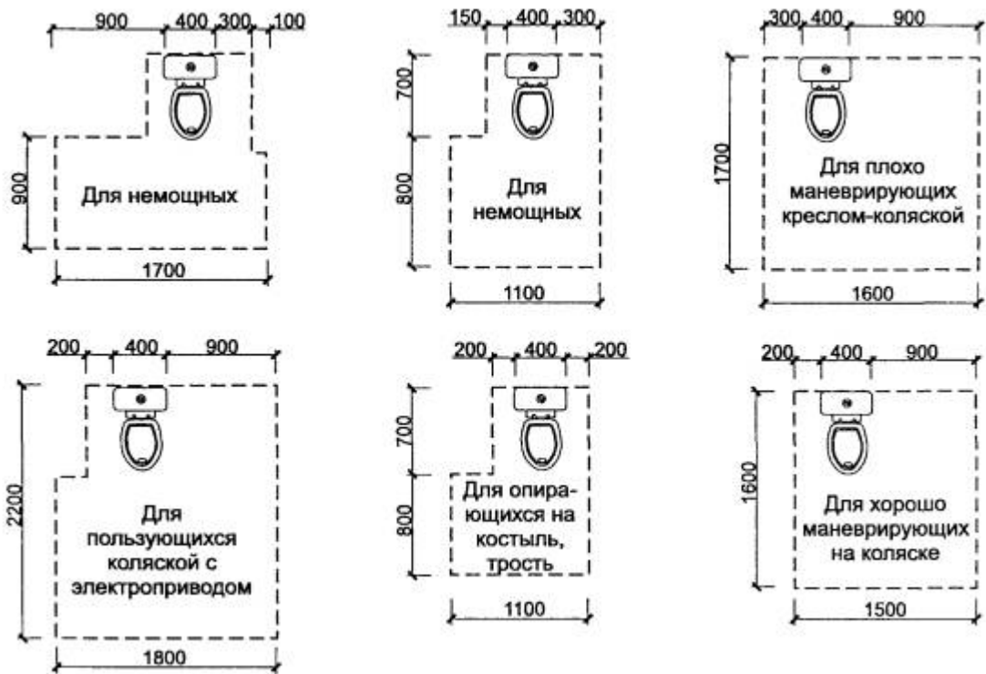
СОВМЕЩЕННЫЕ САУЗЛЫ ДЛЯ ИНВАЛИДОВ, ПОЛЬЗУЮЩИХСЯ КРЕСЛОМ-КОЛЯСКОЙ, ОБОРУДОВАННЫЕ ВАННОЙ
