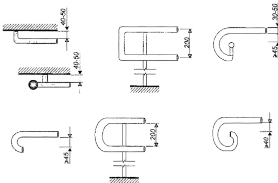
Элементы, фиксирующие окончание поручня
