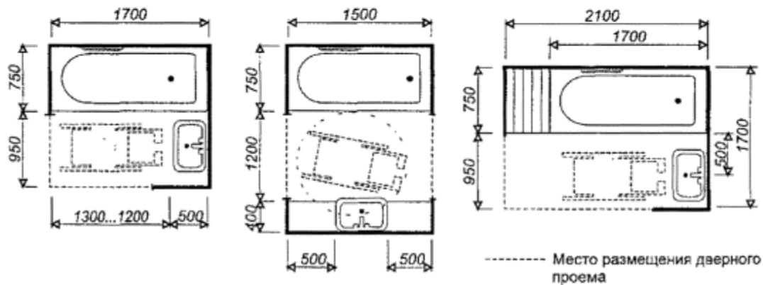
Варианты планировки ванной комнаты
