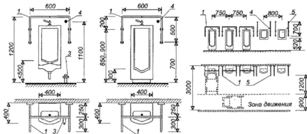
Писсуары для инвалидов
