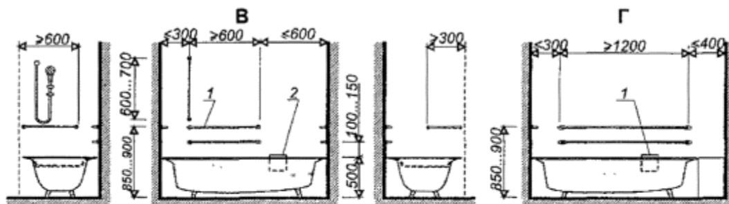
Поручни в кабинах с ванными для "сидячих" (В) и "лежачих" (Г) инвалидов
