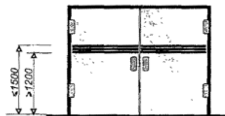
Размещение предупреждающей маркировки на двупольной стеклянной двери
