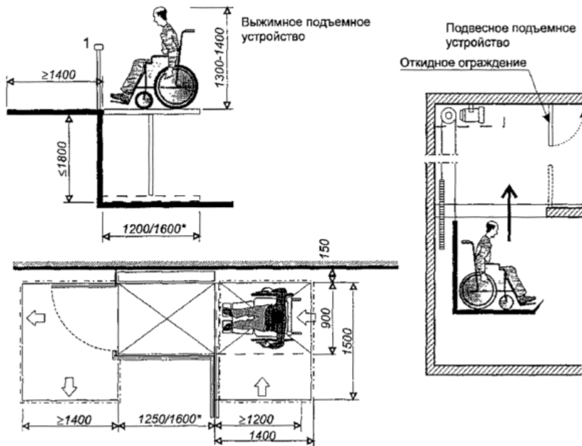
Габариты зоны для установки домашнего лифта и подъемника
