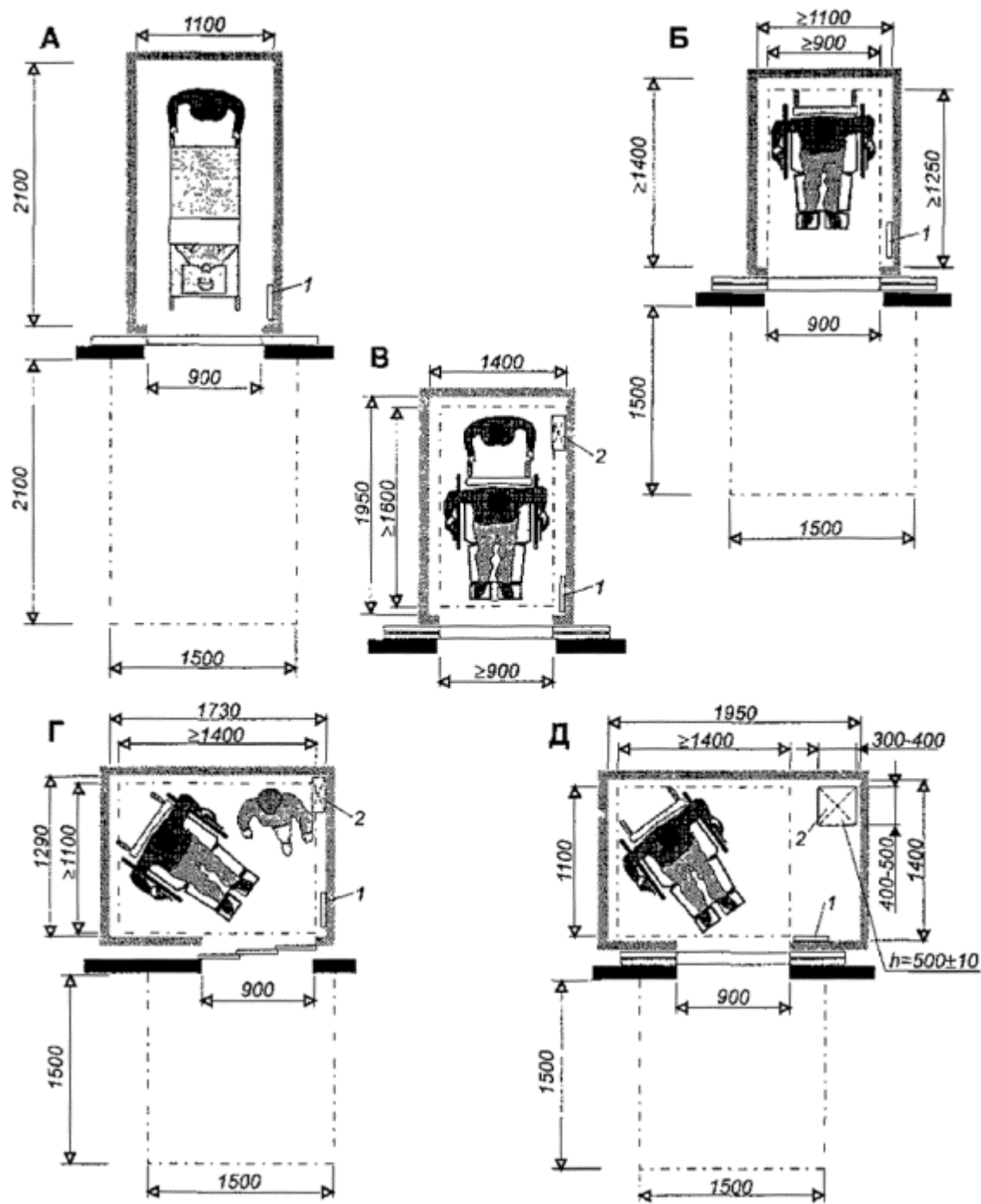
Минимальные внутренние размеры кабины лифта и площадки перед лифтом.
