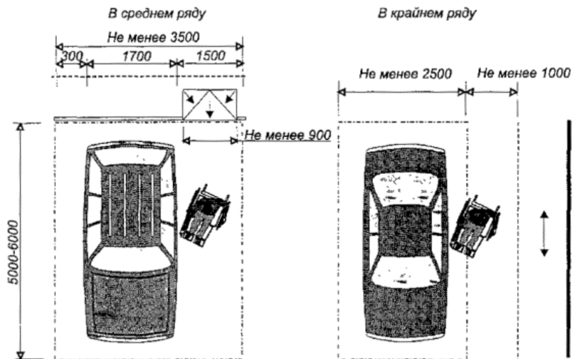
Обозначение мест стоянки автомашин, управляемых инвалидами
