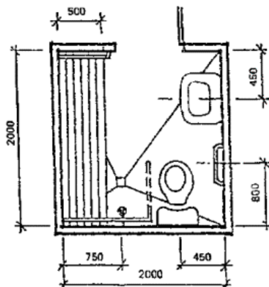
Примеры индивидуальных кабин для переодевания
