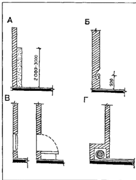
Варианты решения стен спортивных залов
