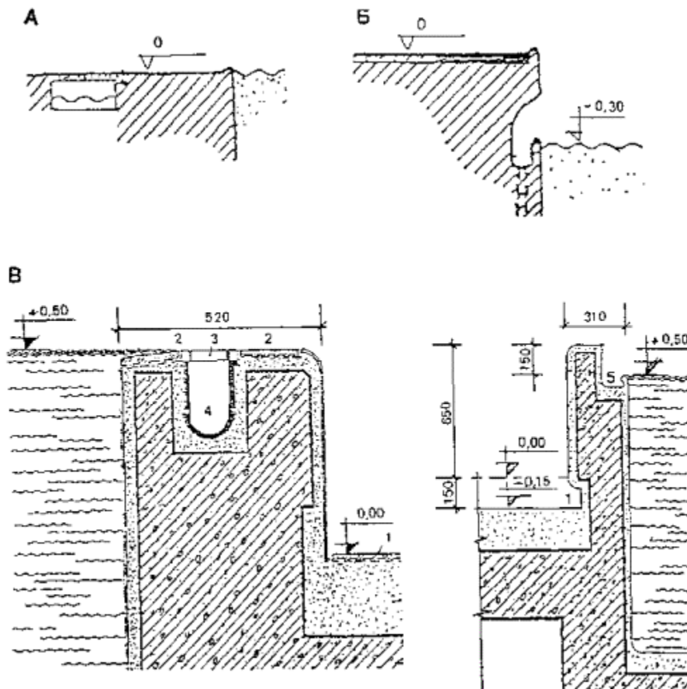
Детали решения бортов ванн бассейнов
