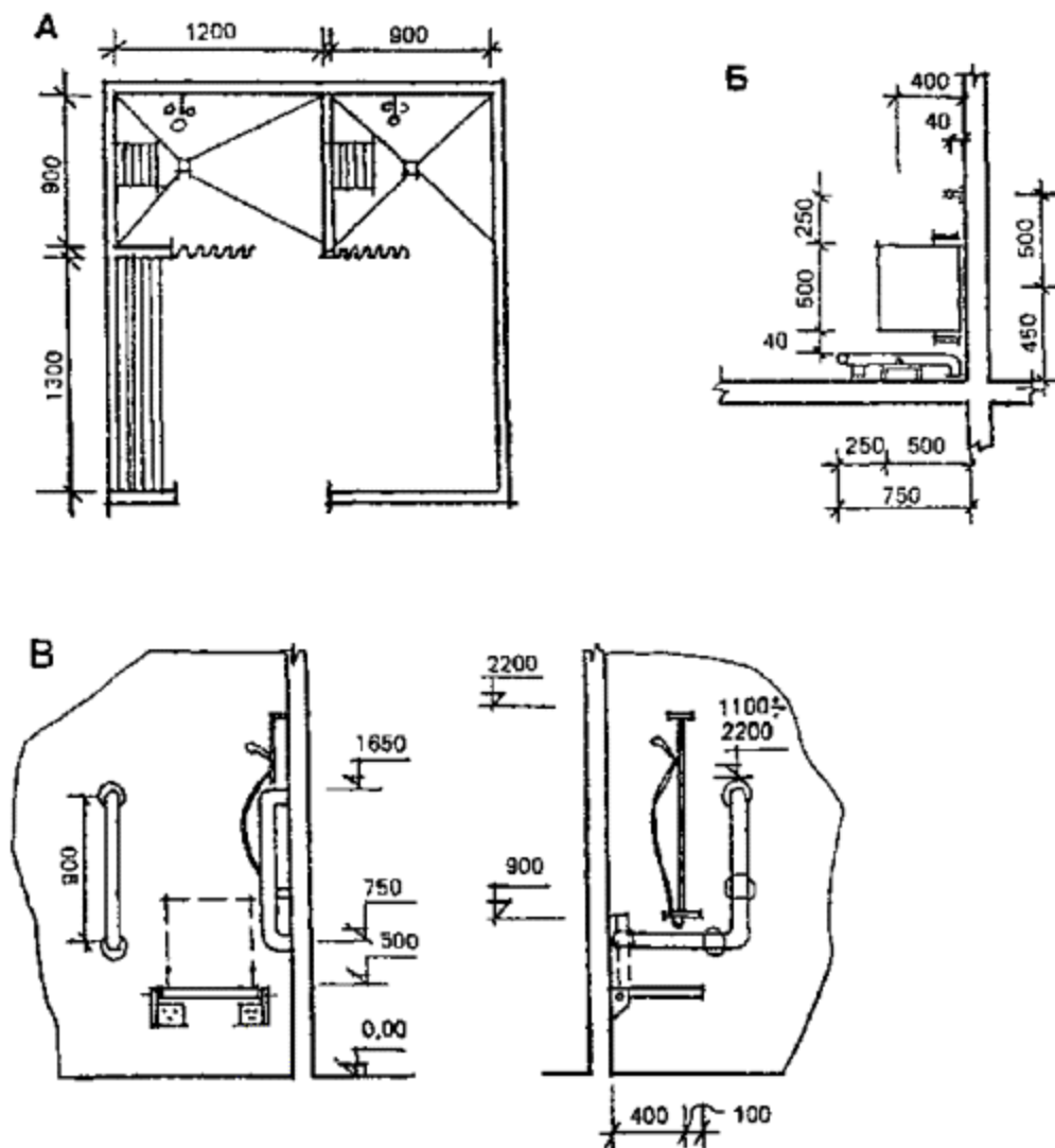
Схемы индивидуальных душевых кабин
