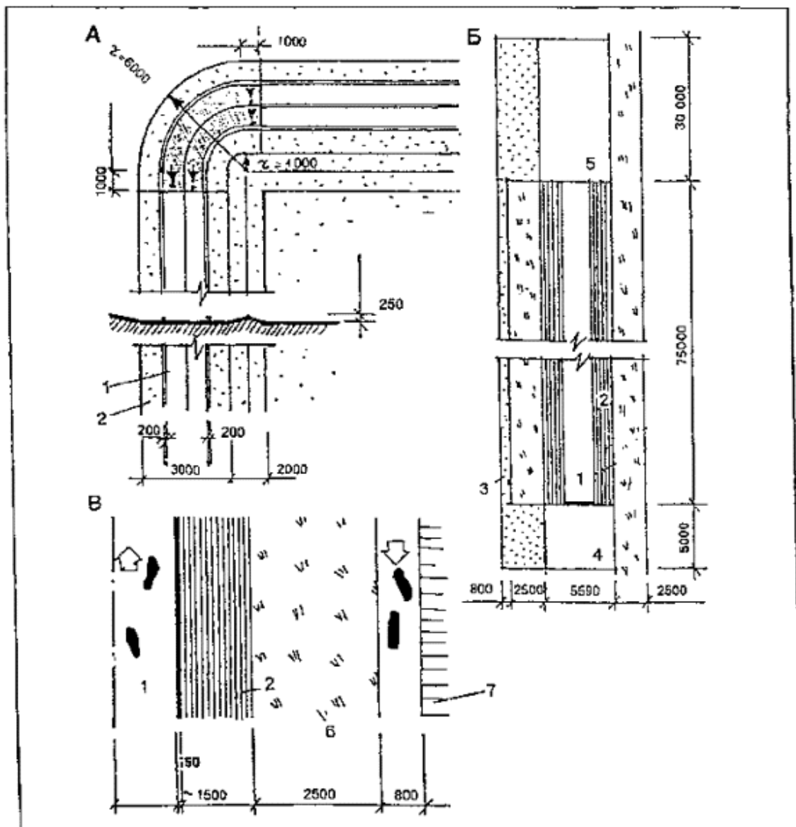
Фрагменты легкоатлетических дорожек
