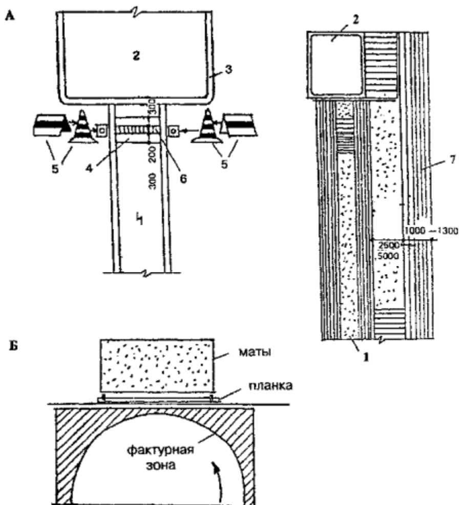
Схема организации места для прыжков для инвалидов с ДЗ
