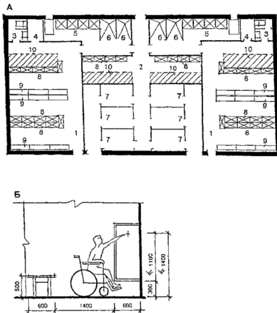
Блок раздевальных и душевых при ванне размером 16,6×8 м
