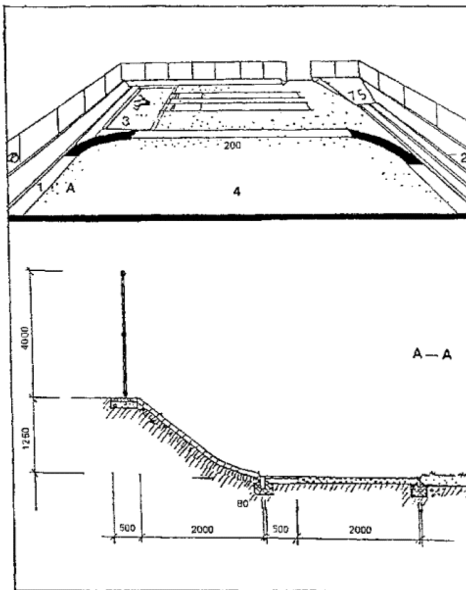
Площадка для занятий легкой атлетикой
