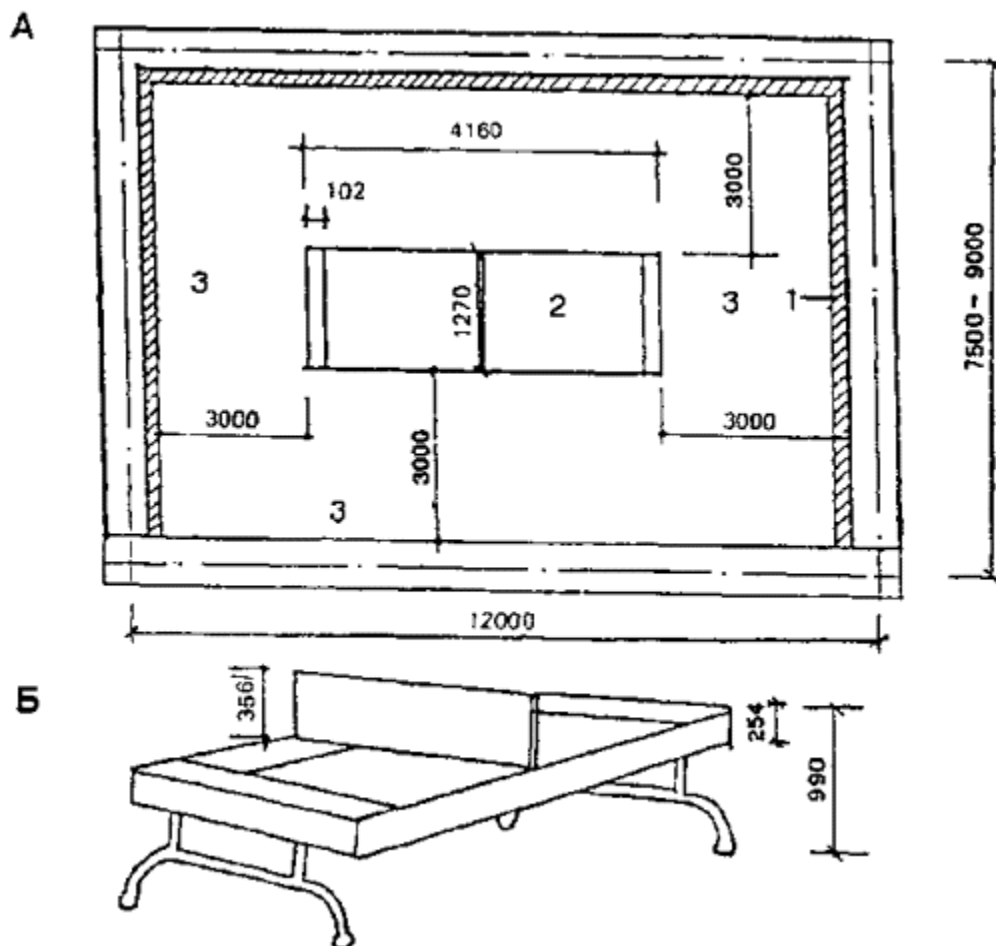
Схема зала для игры в шоу-даун
